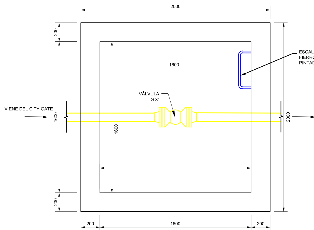
VISTA EN PLANTA (ESCALA 1:20)
