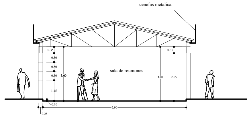
CORTE TRANSVERSAL SALA DE REUNIONES
