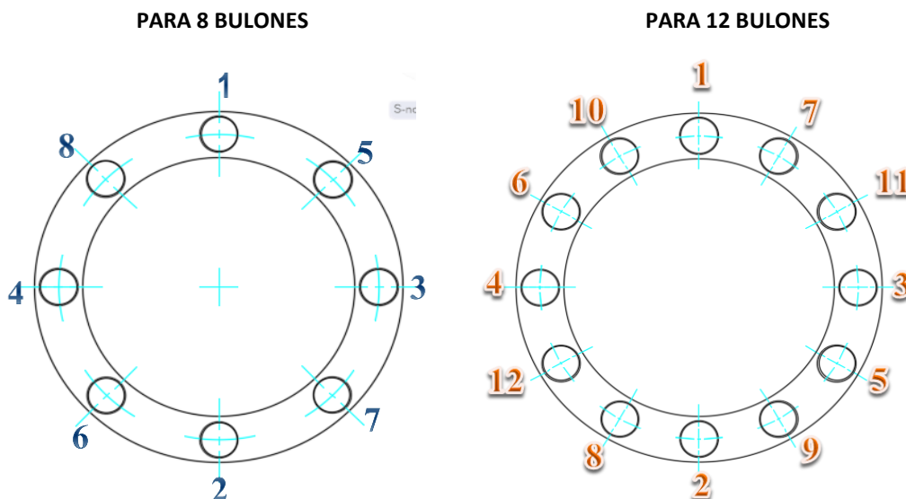
Gráfico 1 SECUENCIA DE AJUSTE DE ESPARRAGOS
