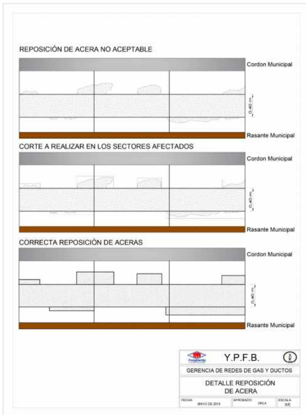
FIGURA 4. REPOSICIÓN Y AFINADO DE ACERAS Y/O CUNETAS
