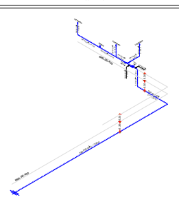
ISOMETRIA SISTEMA DE AGUA POTABLE AMPLIACIONES COMEDOR - LAVANDERIA ESCALA 1:10
