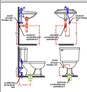
DETALLE DE SALIDAS DE AGUA Y DESAGUE EN SANITARIOS EN ESCALA
