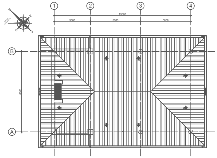
PLANTA CUBIERTA ESCALA: 1/75
