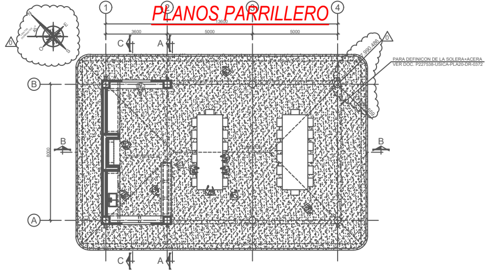
PLANTA BAJA ESCALA: 1/75
