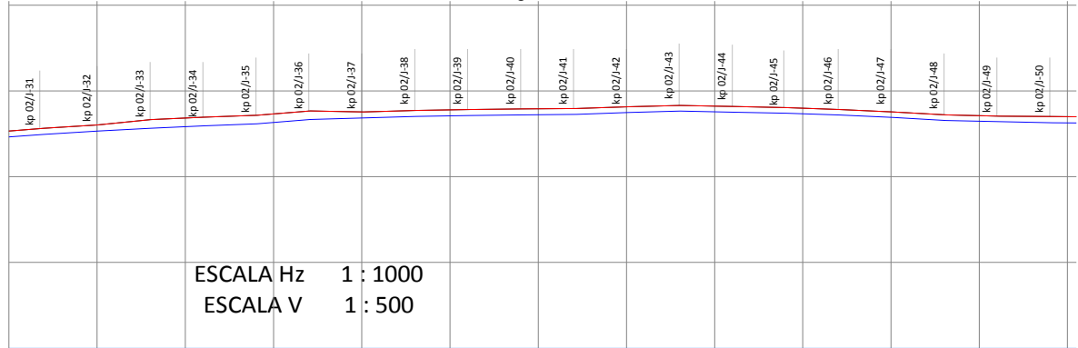
Gráfico 2. Perfil longitudinal.
