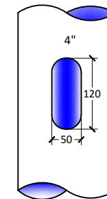
DETALLE DE OVALO PARA ENTRADA DE DUCTO
