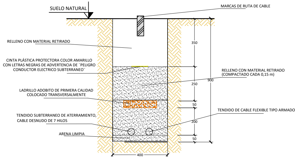
CORTE A-A
