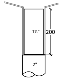
DETALLE DE MARCO DE VENTANILLA DE INSPECCION
