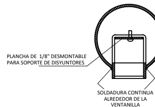
CORTE A-A
