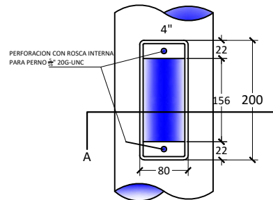
DETALLE DE MARCO DE VENTANILLA DE INSPECCION
