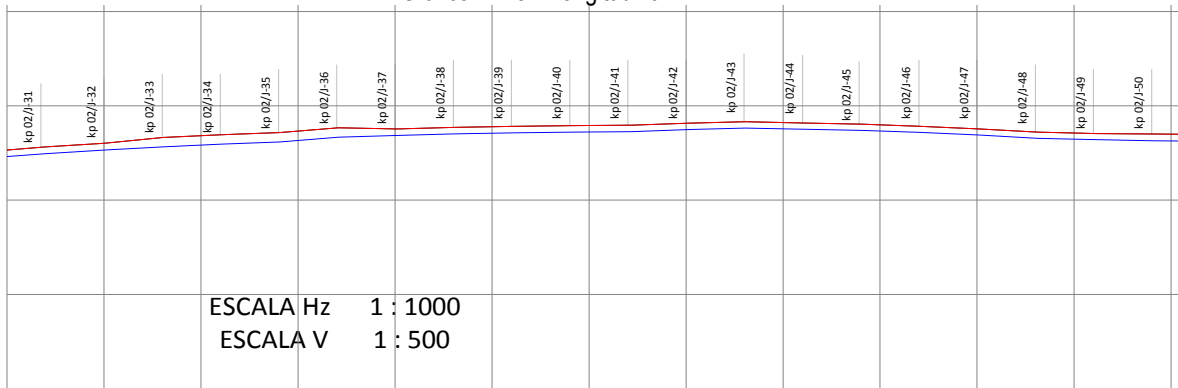
Grafico 2. Perfil longitudinal.
