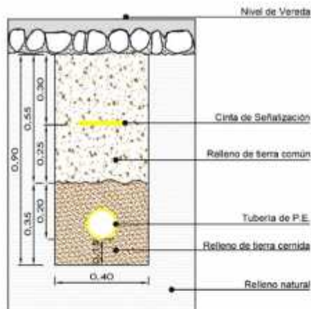
VISTA - CORTE RELLENO DE ZANJA EN VEREDA PARA LINEA DE TUBERIA DE P.E. (Ø=40, 63, 90 MM)
