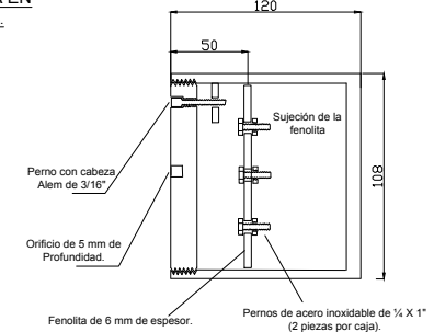
Detalle A
