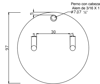
Detalle A
