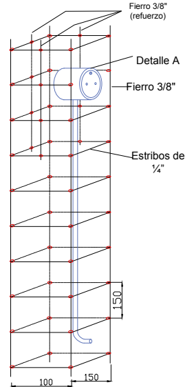
Conexionado
