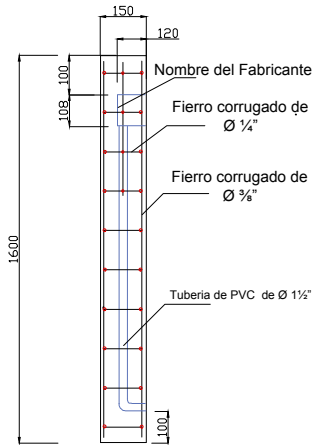
Vista lateral
