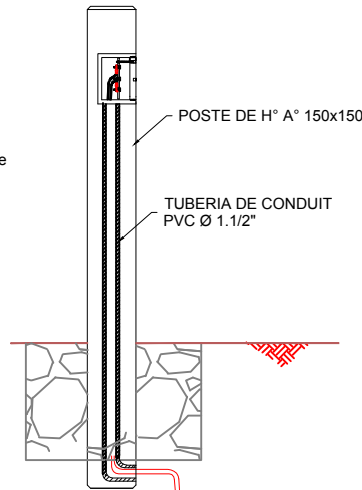
Conexionado
