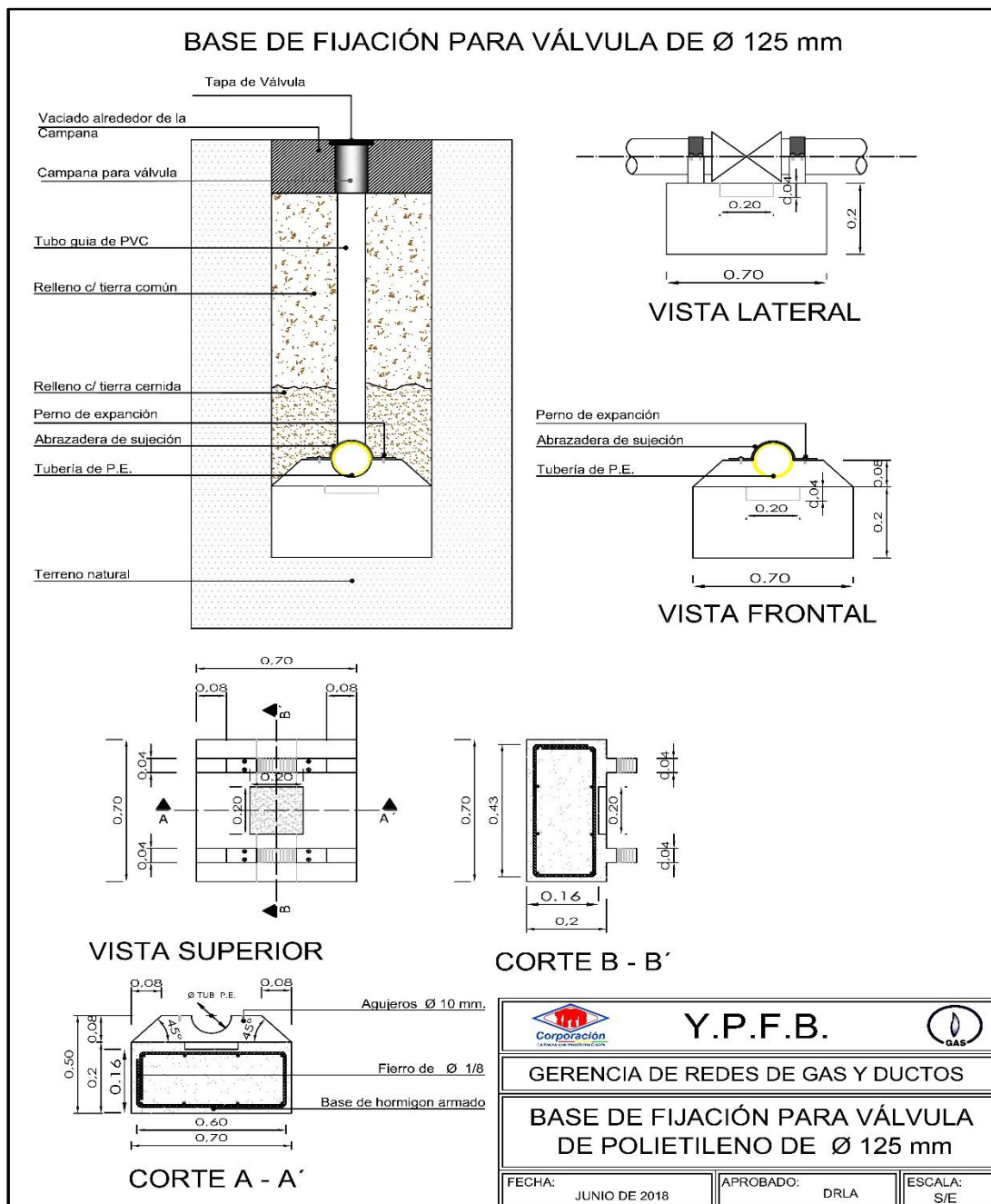
FIGURA 9. DETALLE DE LA BASE DE FIJACIÓN DE VÁLVULA DE P.E. 125 MM
