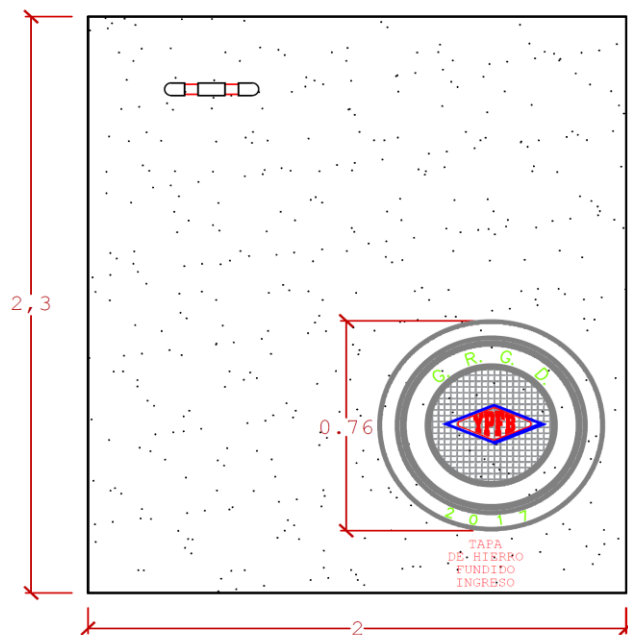
VISTA EN PLANTA LOSA
