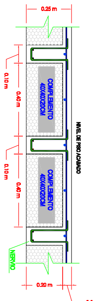
DETALLE DE SECCION TRANSVERSAL DE LOSA ENTERRADA DE HPA®
