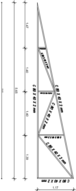
DETALLE DE CERCHA TIPO ADMINISTRACION
